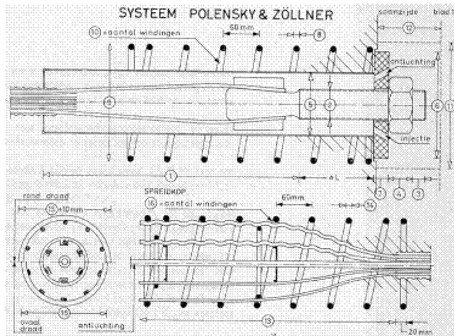
Figuur B3-5: Spanbare -en blinde verankering
