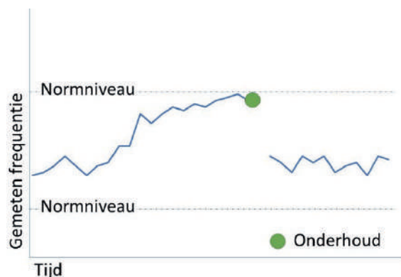
PREVENTIEF ONDERHOUD O.B.V. DETECTIEMETING
