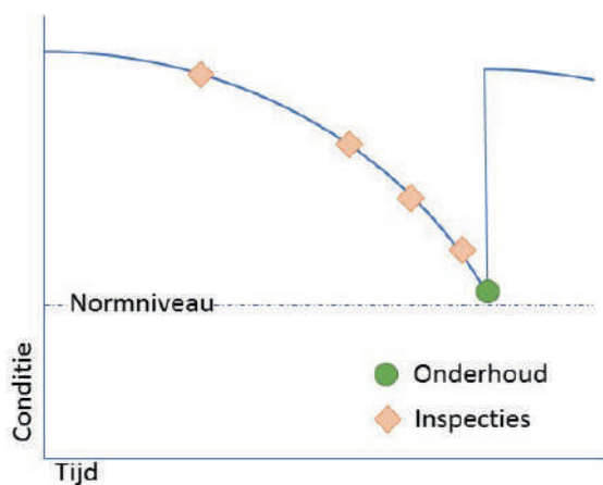
TAO DEGRADATIECURVE
