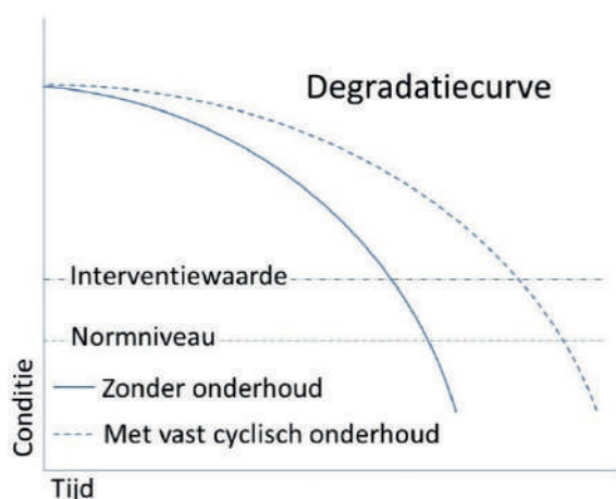
VERSCHUIVING DEGRADATIECURVE
